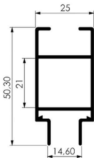
MONTANTE CENTRAL S/ BAGUETE
