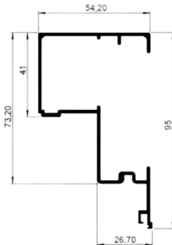
COLUNA LATERAL FACHADA 41MM
