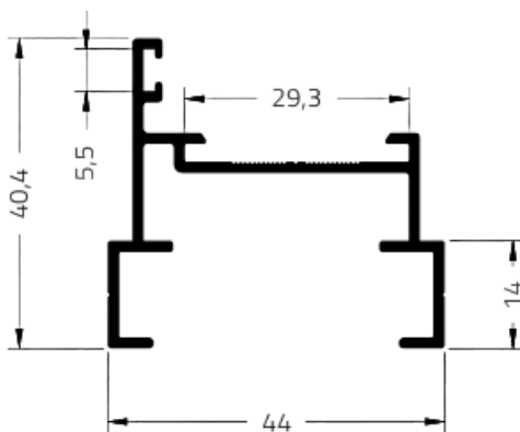
CAIXILHO PORTA GIRO GOLD
