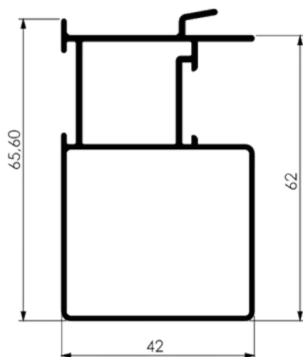
MÃO AMIGA DE PORTA INT. COM BAGUETE
