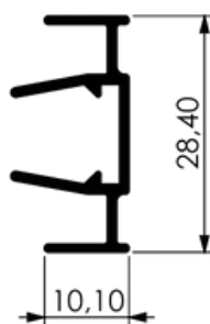
LATERAL (MATA JUNTA)
