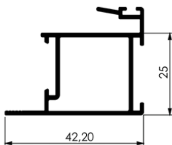
MONTANTE MÃO AMIGA EXTERNO
