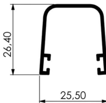
QUEBRA VENTO
