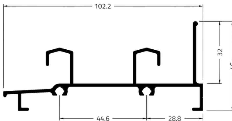
TRILHO INFERIOR LINHA GOLD
