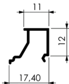
BAGUETE PARA LINHA SUPREMA
