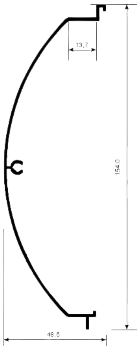
TAMPA INTERNA JANELA INTEGRADA
