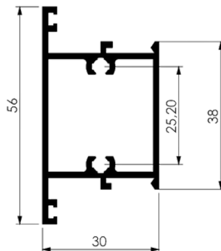
TRAVESSA L30
