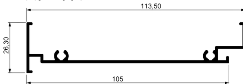
SUPERIOR DA CAIXA INTEGRADA
