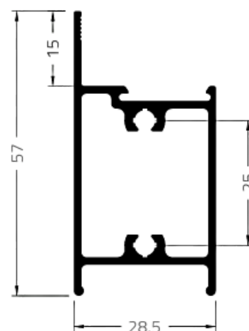
MONTANTE DA FOLHA
