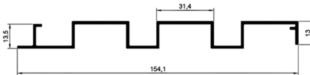
LAMBRI RIPADO
