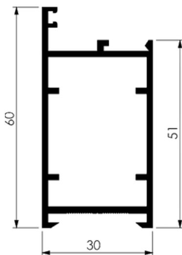
MONTANTE 60MM L30
