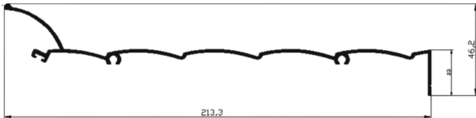
TAMPA EXTERNA INTEGRADA
