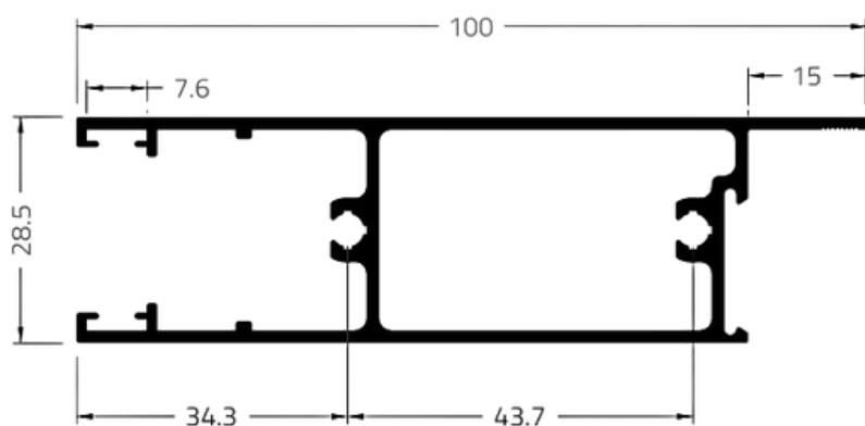
TRAVESSA INFERIOR FOLHA GOLD
