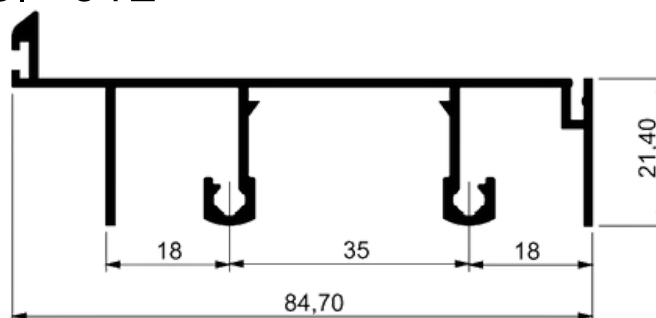
TRILHO SUPERIOR INTEGRADA
