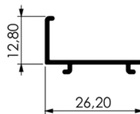
PINGADEIRA DA FOLHA
