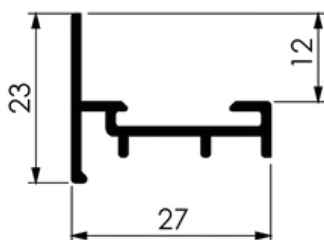
CADEIRINHA FIXO BASCULANTE
