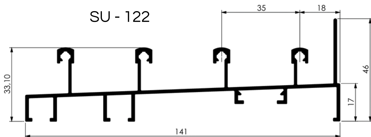
TRILHO INFERIOR 4 FOLHAS
