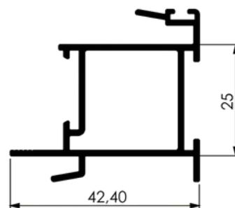
MONTANTE MÃO AMIGA LADO ESQUERDO
