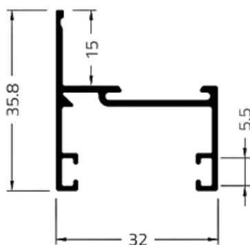
MARCO LATERAL LINHA GOLD
