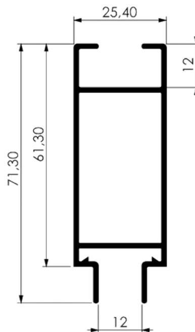
MONTANTE 4 FOLHAS COM BAGUETE
