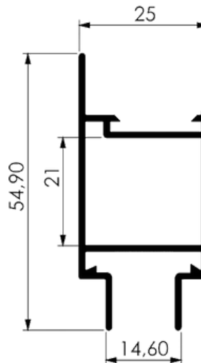
MONTANTE CENTRAL COM BAGUETE
