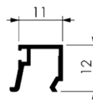
BAGUETE L25
