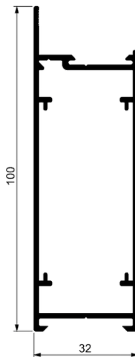
MONTANTE LINHA GOLD 100MM
