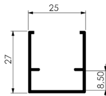
MARCO DA FOLHA
