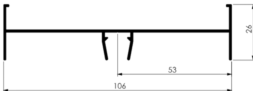
MARCO LATERAL 3 PLANOS
