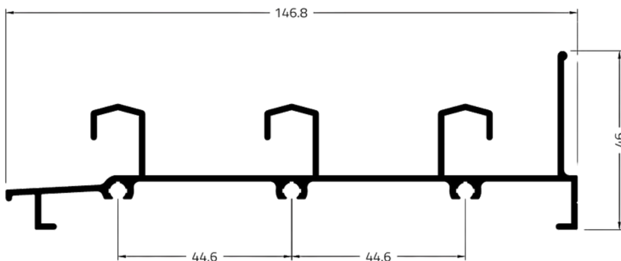
TRILHO INFERIOR 3 PLANOS GOLD
