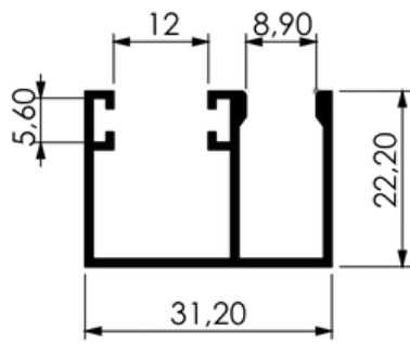
TRILHO INFERIOR V 8MM
