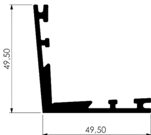
CANTONEIRA LINHA SUPREMA/25
