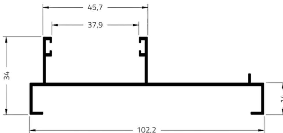
MONTANTE LATERAL GOLD
