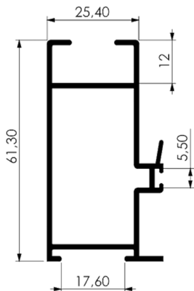
MONTANTE PORTA SEM BAGUETE
