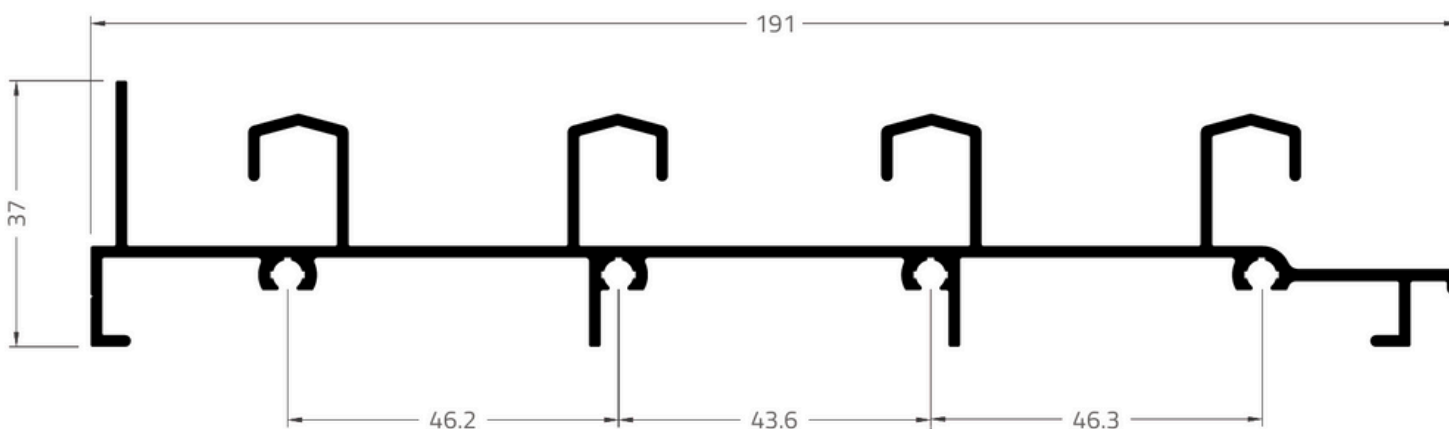
TRILHO DE BAIXO 4 PLANOS GOLD
