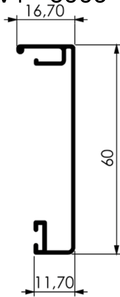
CAPA COM ESCOVA (60MM)
