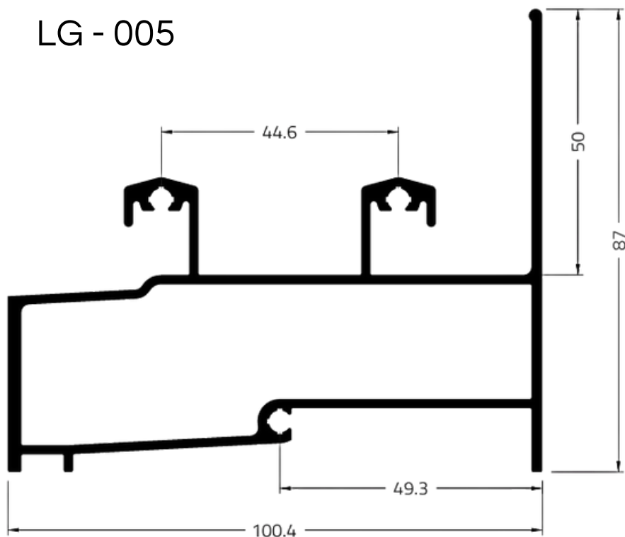
TRILHO INF. 2 PLANOS C/REFORCO GOLD
