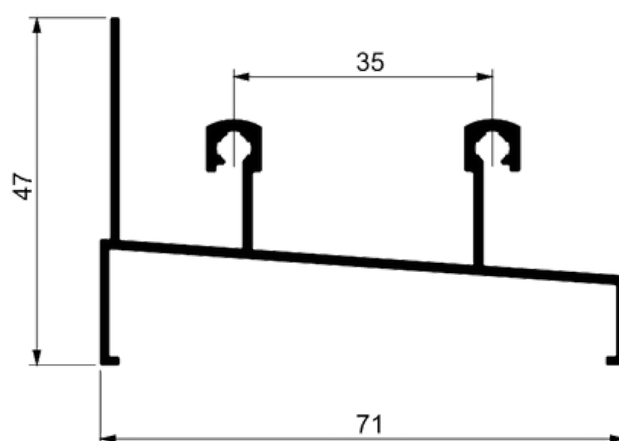
TRILHO INFERIOR
