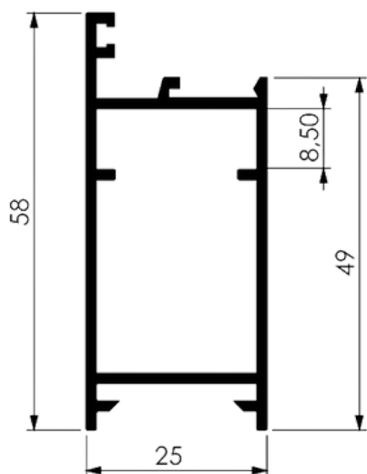
MONTANTE PARA PORTA L25
