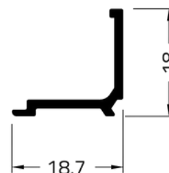
BAGUETE PARA VIDRO DUPLO GOLD
