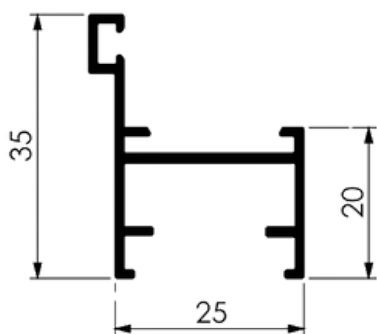
CAIXILHO MAXIM-AR
