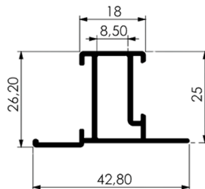
MONTANTE FOLHA MAXIM-AR
