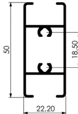
TRAVESSA FOLHA S/ BAGUETE
