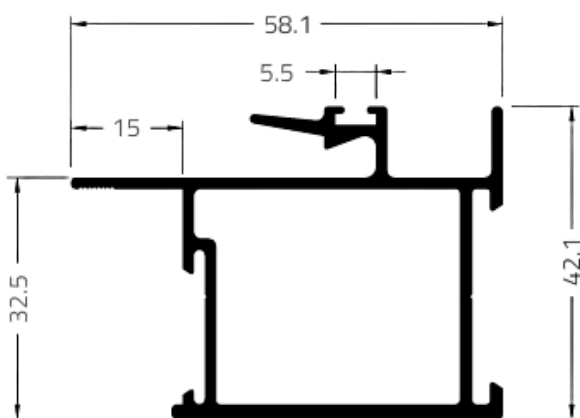
MONTANTE MAO AMIGO INTERNO GOLD
