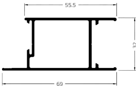
MONTANTE DA FOLHA GOLD
