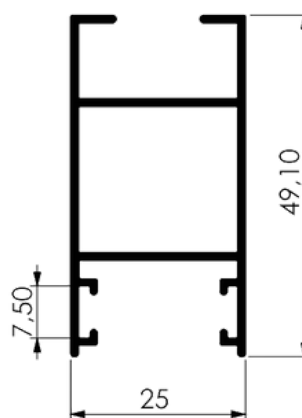
MONTANTE DA FOLHA S/BAGUETE
