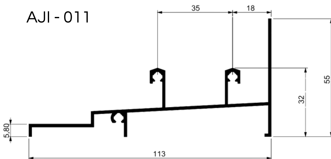
TRILHO INFERIOR INTEGRADA
