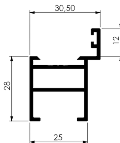
MARCO PARA PORTA L25
