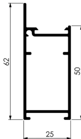
MONTANTE DA FOLHA DE GIRO C BAGUETE
