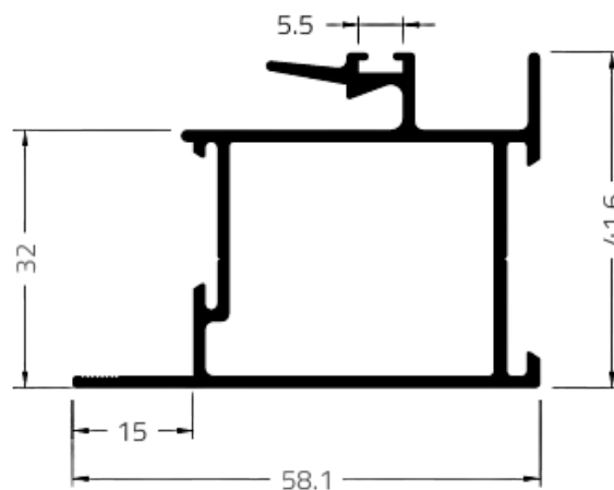
MONTANTE MAO AMIGO EXTERNO GOLD
