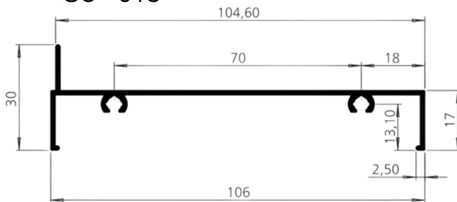
MARCO SUPERIOR 3 PLANOS
