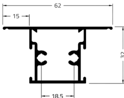
TRAVESSA LINHA GOLD
