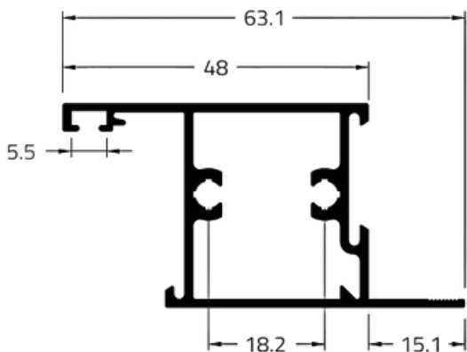
TRAVESSA INVERSOR DE BAGUETE
