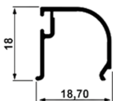
BAGUETE REDONDO (MEDIO)
