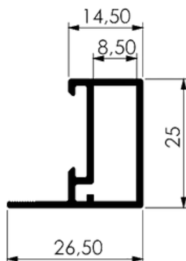
MONTANTE DA FOLHA
