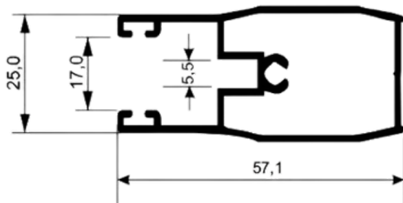
GUIA LATERAL DA PERSIANA
