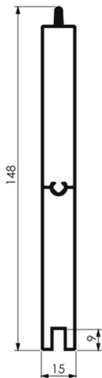
LAMBRI DUPLO 150MM
