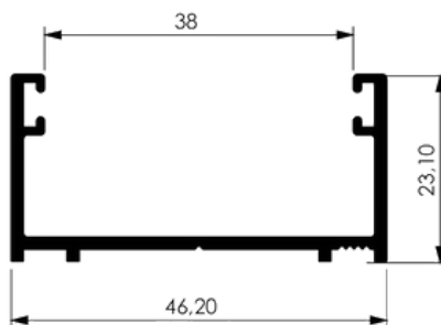
BATENTE LINHA GOLD
