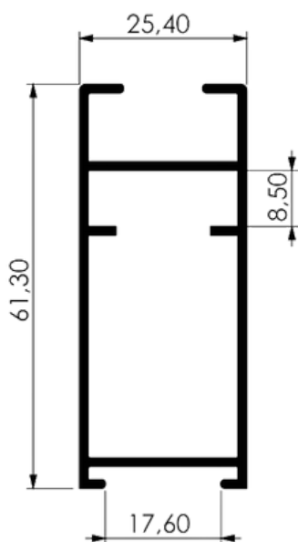
FOLHA LATERAL SUPREMA S/ BAGUETE
