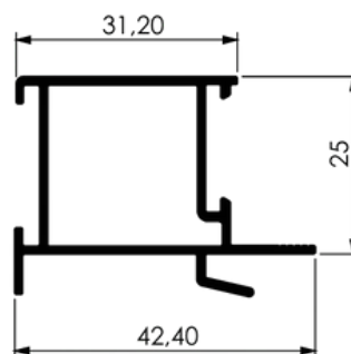
MONTANTE MÃO AMIGA INTERNA C/BAGUETE
