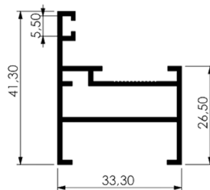
CAIXILHO PORTA GIRO
