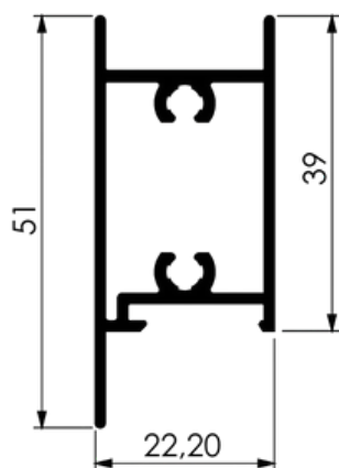
TRAVESSA DA FOLHA
