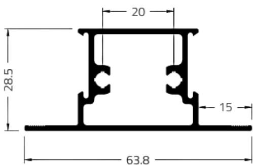
TRAVESSA DA FOLHA GOLD
