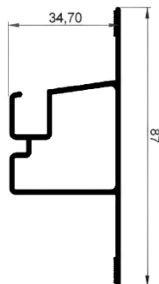
TRAVESSA PARA FACHADA
