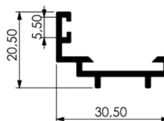
BATENTE P/ PORTA DE ABRIR L25
