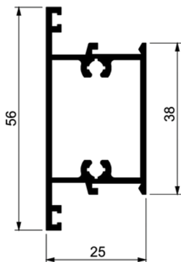
MONTANTE DA TRAVESSA L25
