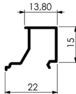
BAGUETE MAIOR P/ LINHA SUPREMA
