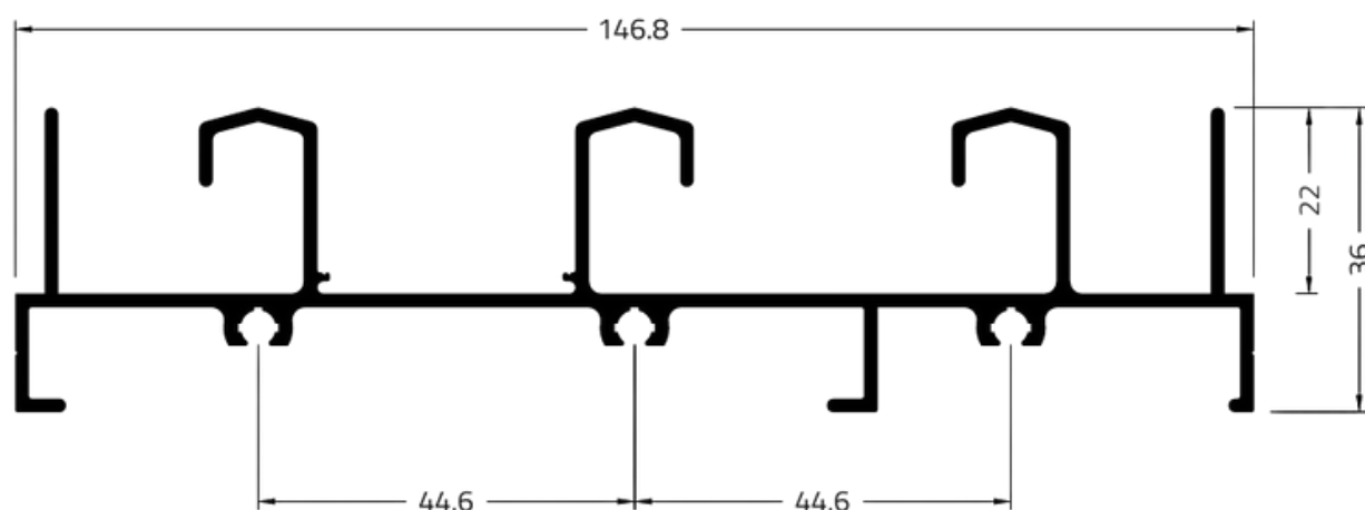
TRILHO SUPERIOR 3 PLANOS GOLD
