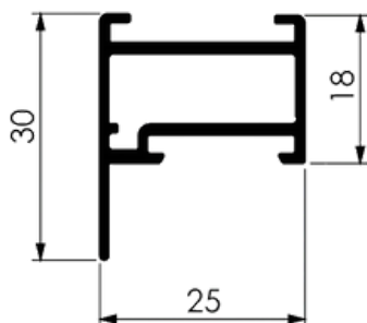
TRAVESSA SUPERIOR FOLHA 45
