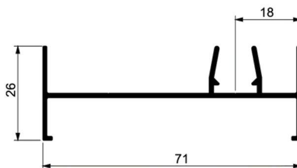
MARCO LATERAL DE CORRER
