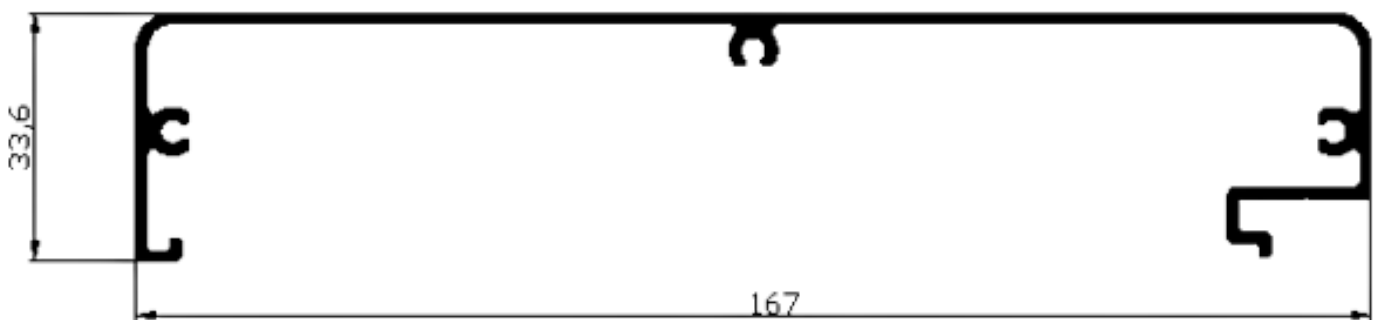
TAMPA INTERNA JANELA INTEGRADA
