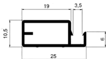
PERFIL P/ TELA MOSQUITEIRO
