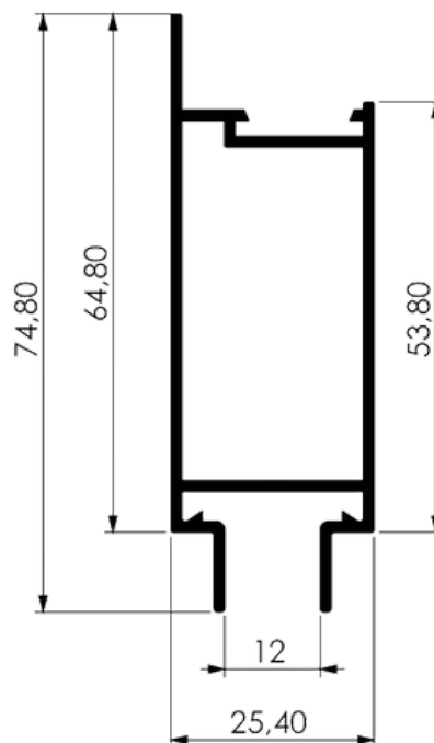
MONTANTE LINHA SUPREMA
