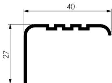
ARREIMATE DE PISO
