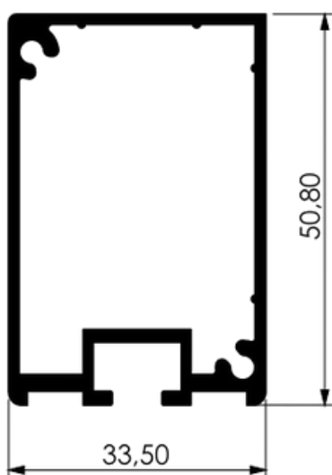
TUBO COLUNA GRADIL PANORAMA
