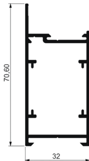
MONTANTE FOLHA GOLD
