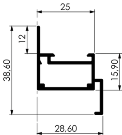
TRAVESSA DA FOLHA
