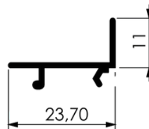
COMPLEMENTO VENEZIANA
