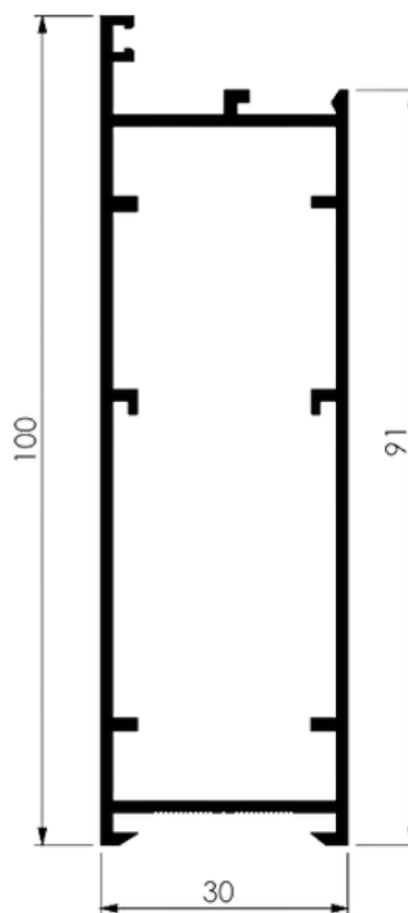
MONTANTE 100MM L30
