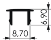
CLICK PARA VT 8MM
