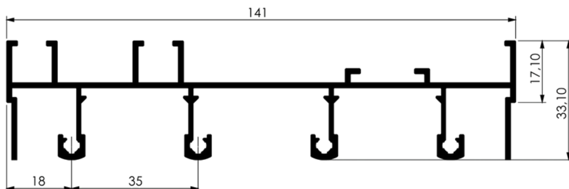
TRILHO SUPERIOR 4 FOLHAS
