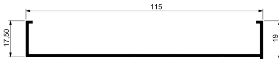
MONTANTE LATERAL INTEGRADA
