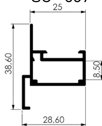
MONTANTE DA FOLHA BASCULANTE
