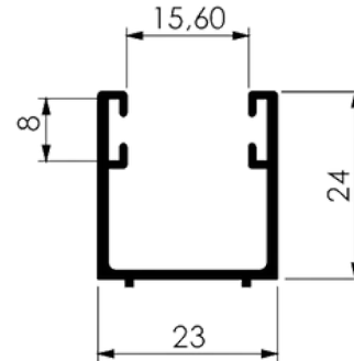
TRILHO INFERIOR SIMPLES V 8MM
