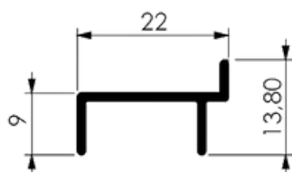
PORTA PALHETA DA L25
