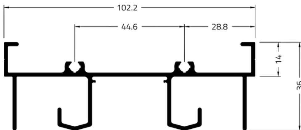
TRILHO SUPERIOR LINHA GOLD
