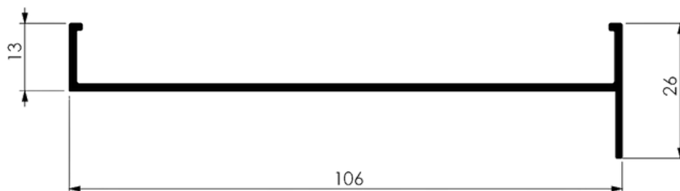
MARCO LATERAL 3 PLANOS
