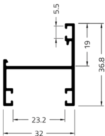
MARCO MAXIM-AR LINHA GOLD
